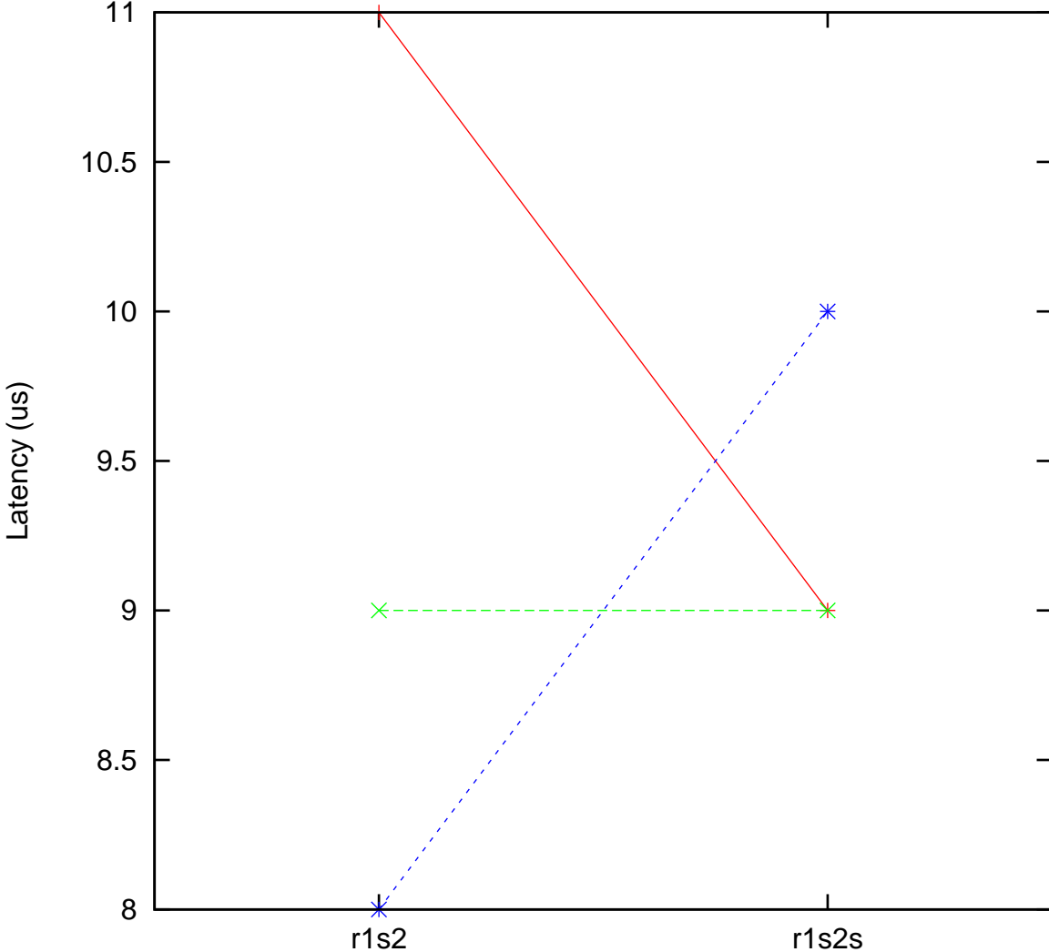
Moderate load maximum latency x86 Intel Xeon E3-1220L V2 200 MHz, Linux 4.4.229-rt200 vs. x86 Intel Xeon E3-1220L V2 200 MHz, Linux 4.4.229-rt200
