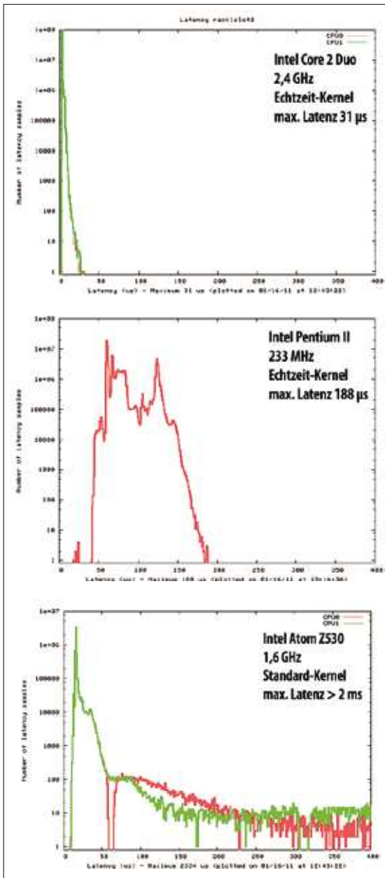
Bild 3. Mit dem Programm Cyclictest gewonnene Latenz-Plots. Zur besseren Vergleichbarkeit wurde in allen drei Plots die gleiche Skalierung gewählt. Grüne und rote Linien stehen für die verschiedenen Cores – oben und unten jeweils ein Dual-Core-Prozessor.
