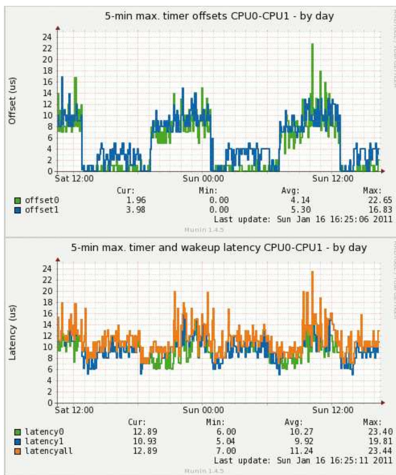
▮ Bild 1. Langzeit-Registrierung von Systemdaten und Echtzeit-Parametern mit Hilfe von Munin. Die im 5-Minuten-Takt registrierten Werte zeigen eine normale Reaktion der Latenzen auf die verschiedenen Lastbedingungen.
