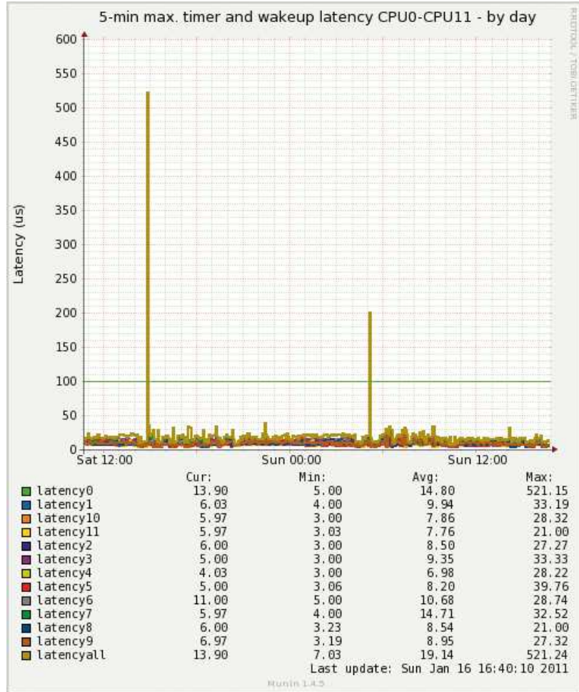
Bild 2. Registrierung von zwei unerwarteten Latenzen, deren Ursache analysiert und beseitigt werden muss.
